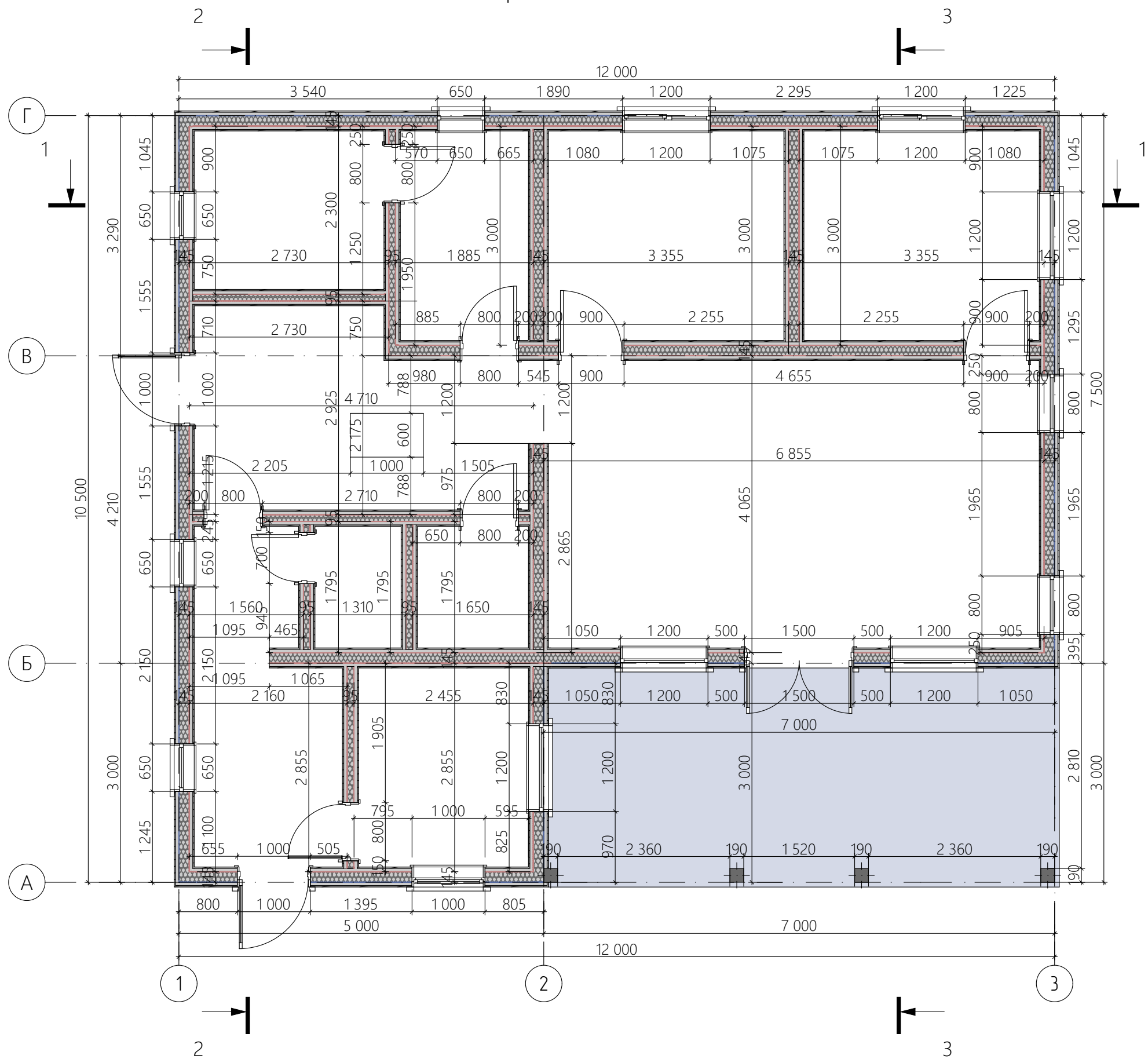
Размерный план 1 этажа
